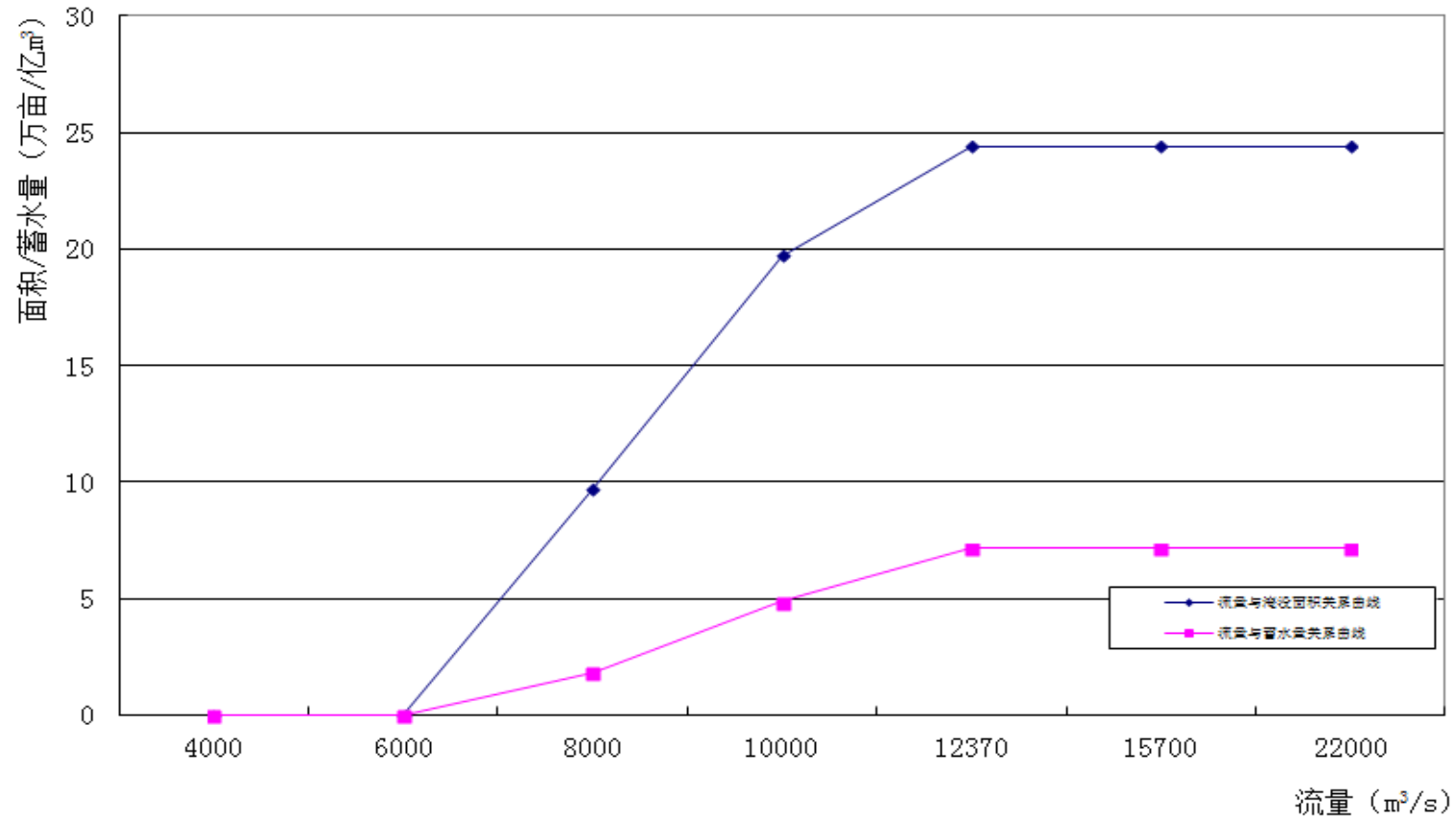
平阴县黄河滩区流量、面积、蓄水量曲线图
